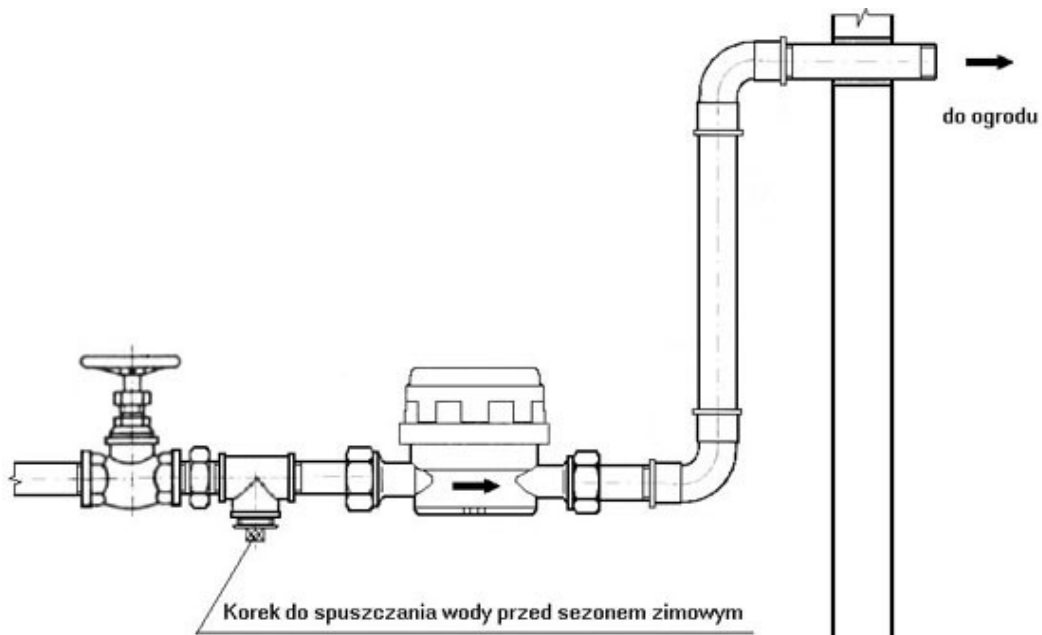
Przykładowa zabudowa podlicznika do podlewania ogrodu
